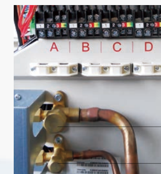
Centrální uzavírací ventil
